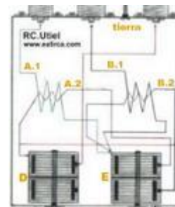
Acoplador Fig.52
